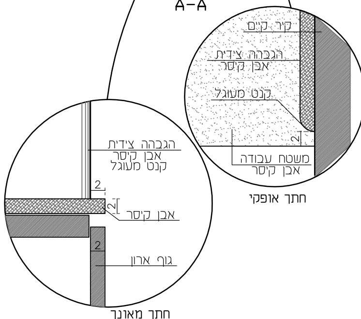
A-A
